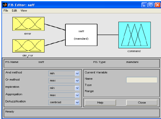
Fig. 7 FIS EDITOR
